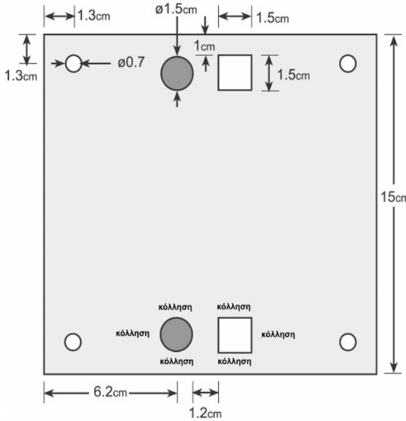
Βάση Στόχου (σχέδιο)
