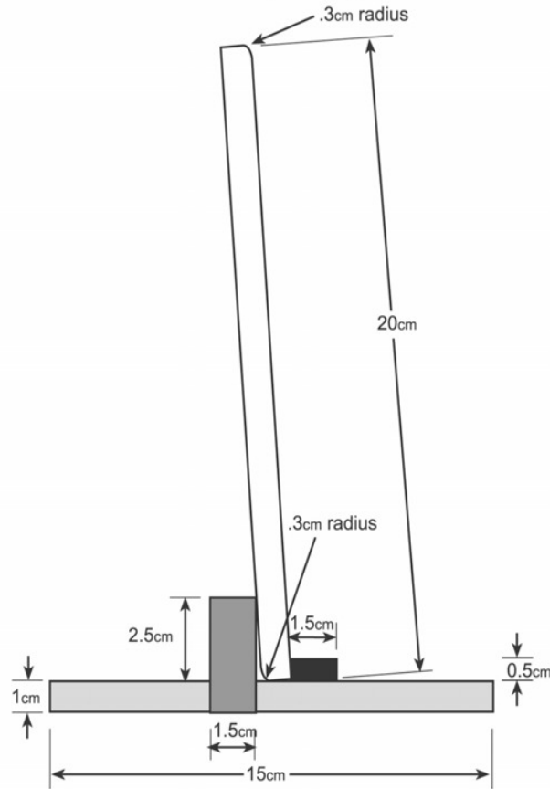
Πλήρης Στόχος Πλάγια Όψη
